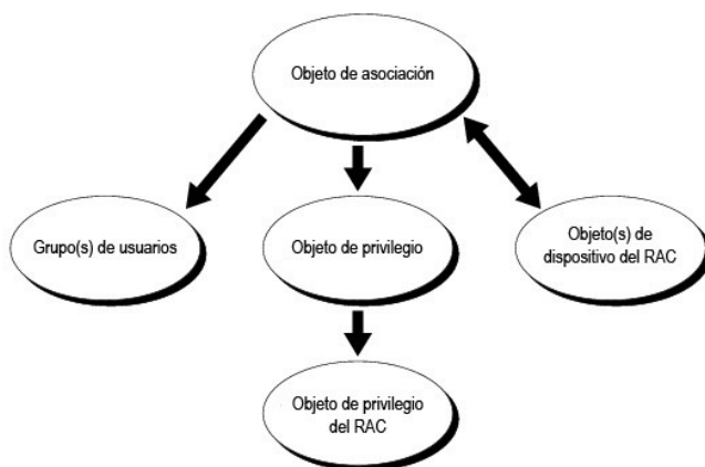
Figura 6-1. Configuración típica de los objetos de Active Directory
